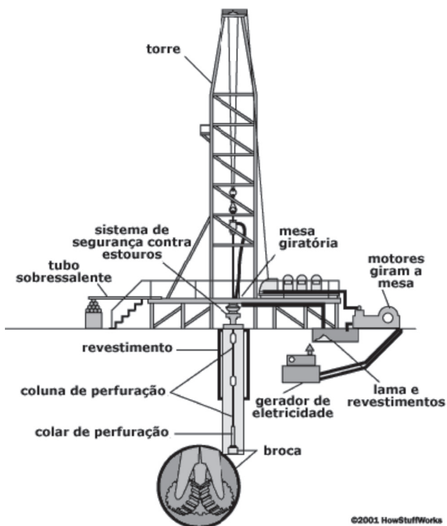
FIGURA 34. Sondagem rotativa
